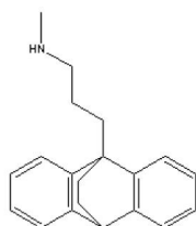
2. Maprotiline (I.S.)
